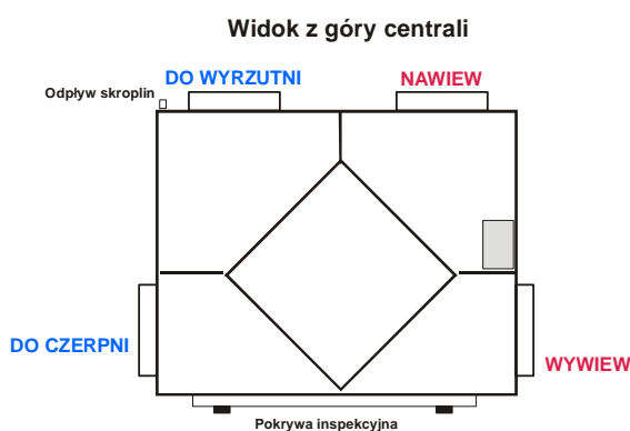
Wykonanie lewe (MISTRAL P) z wylotami od tyłu
